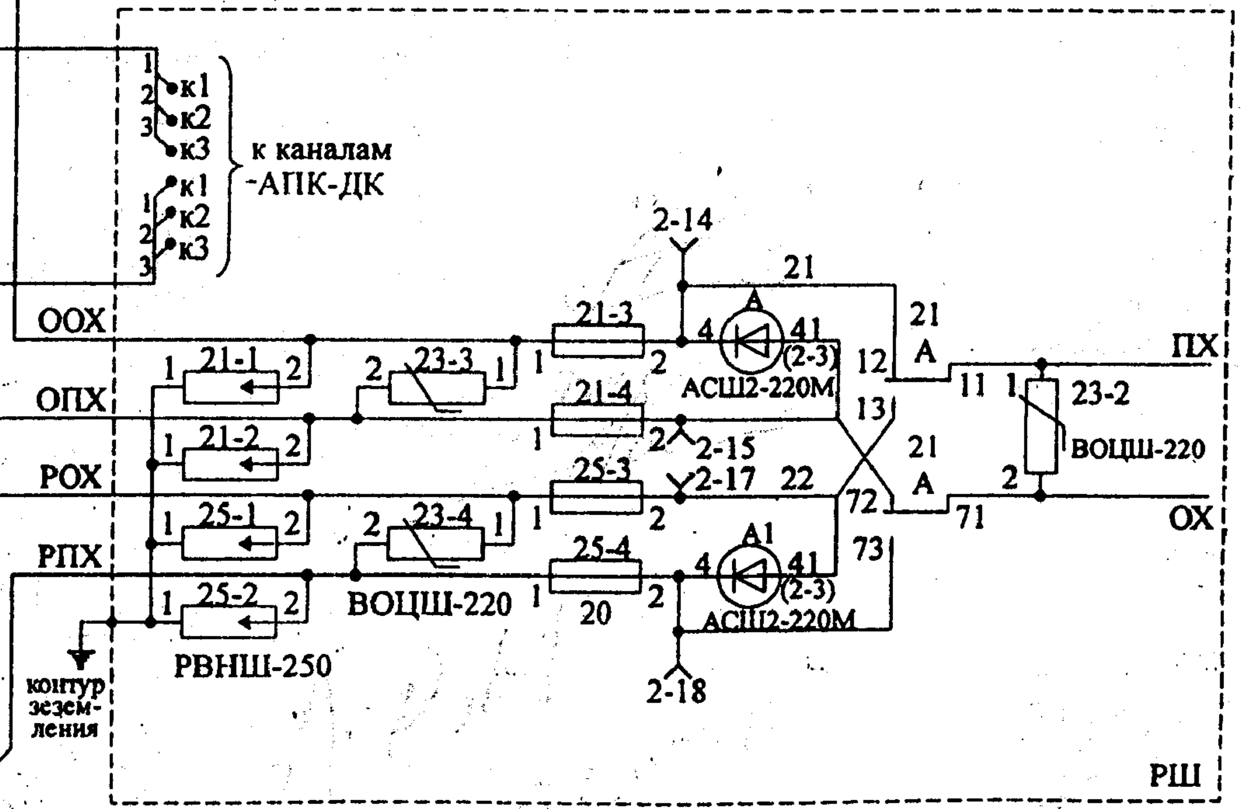
Схема включения кабельных ящиков с аппаратурой защиты 3Ф-220 по основному и резервному питанию на сигнальных установках автоблокировки.
