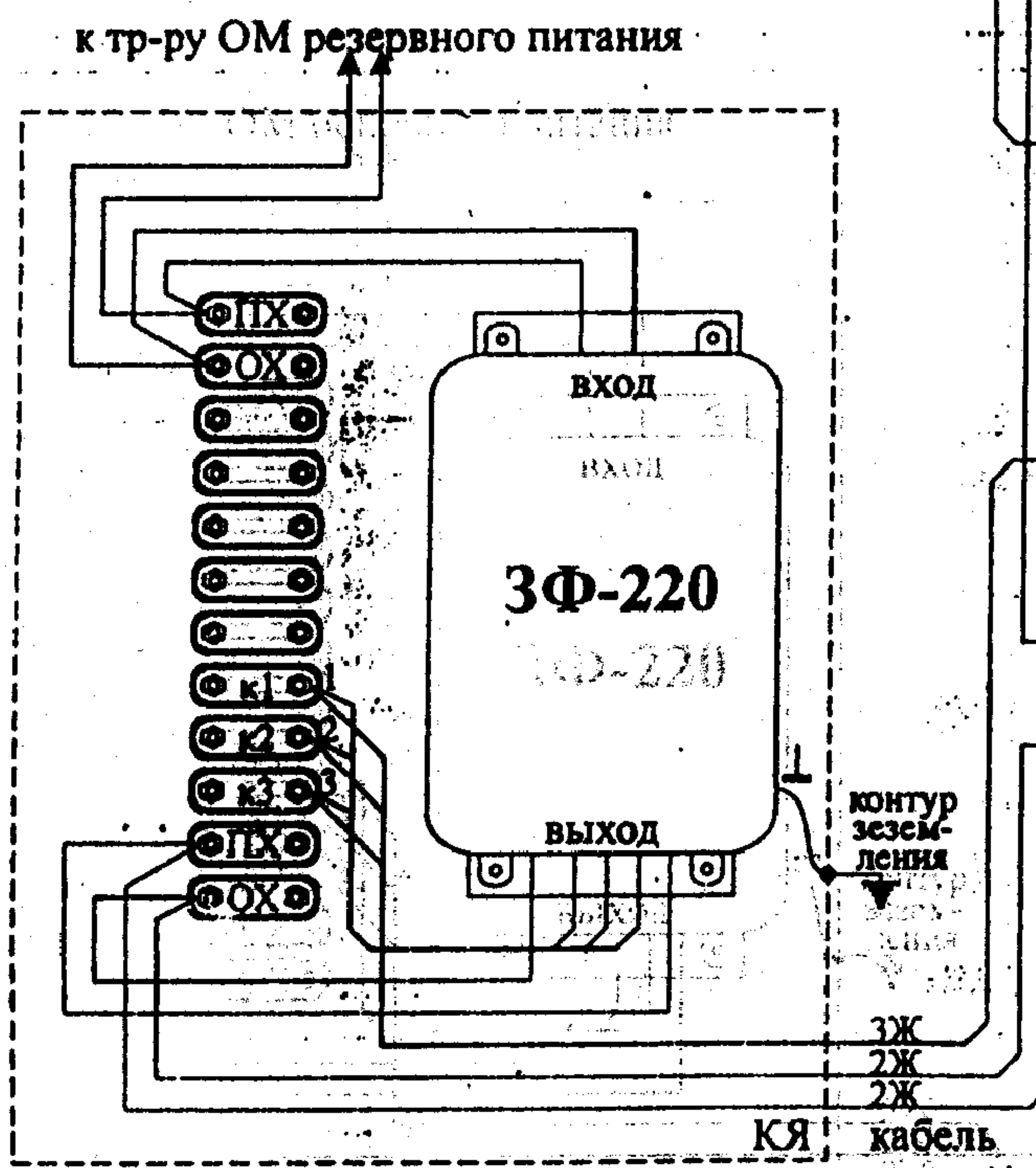
Схема включения кабельных ящиков с аппаратурой защиты 3Ф-220 по основному и резервному питанию на сигнальных установках автоблокировки.
