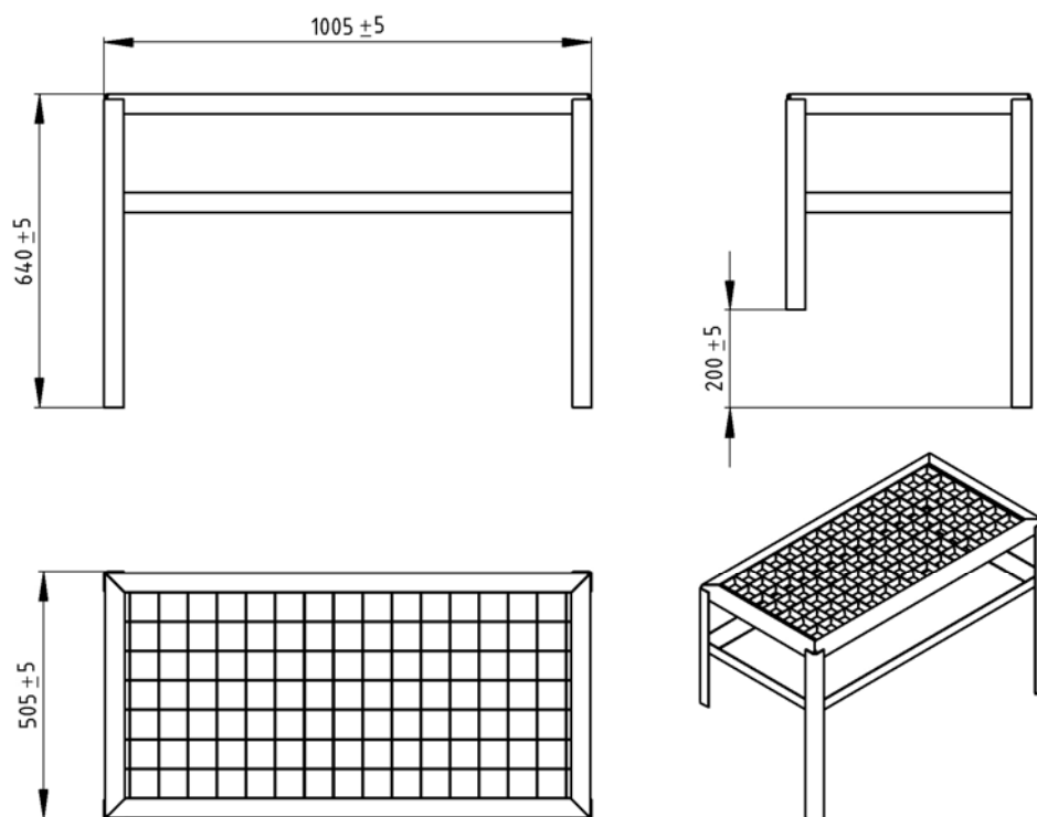
Рисунок А.3 Габаритные размеры площадки шкафа ШРУ-3
