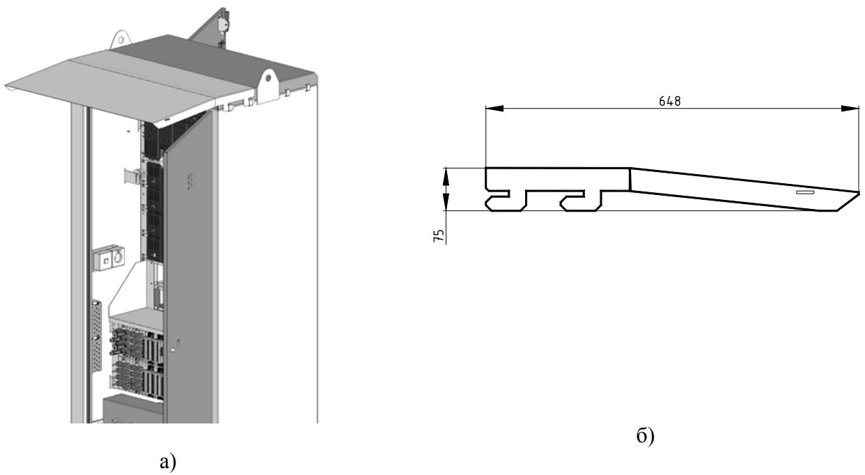
Рисунок А.4. Эскиз установки площадки
