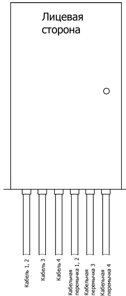
Рисунок А.6. Схема ввода кабелей и кабельных перемычек в аппаратуру защиты БАРЬЕР-АБЧК-2
