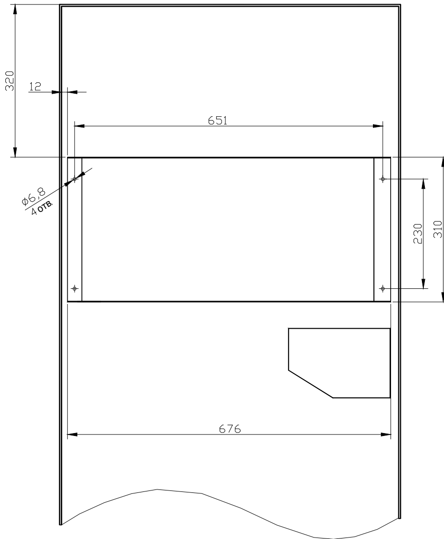
Рисунок А.5. Установка аппаратуры защиты БАРЬЕР-АБЧК-3 на дверь релейного шкафа
