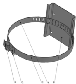
1 – Основание; 2 –пояс; 3 –пластина; 4 – Винт стяжной; 5 – Лепесток. Рисунок 3
