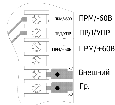
Рисунок 1 – Расположение контактов на клеммной колодке ППУ.
